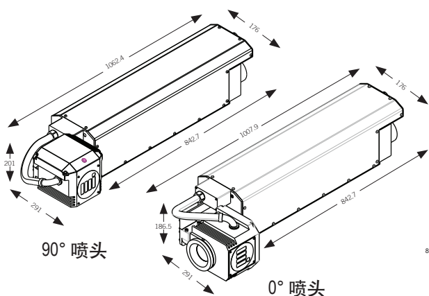
激光打印头
