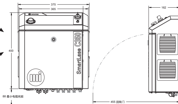
控制器
